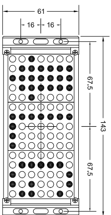
OPTIONAL BRACKET POSITION 'B-B'
